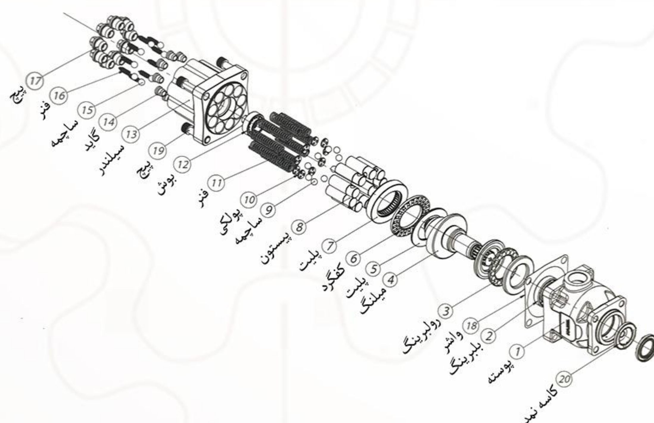
نمای انفجاری
